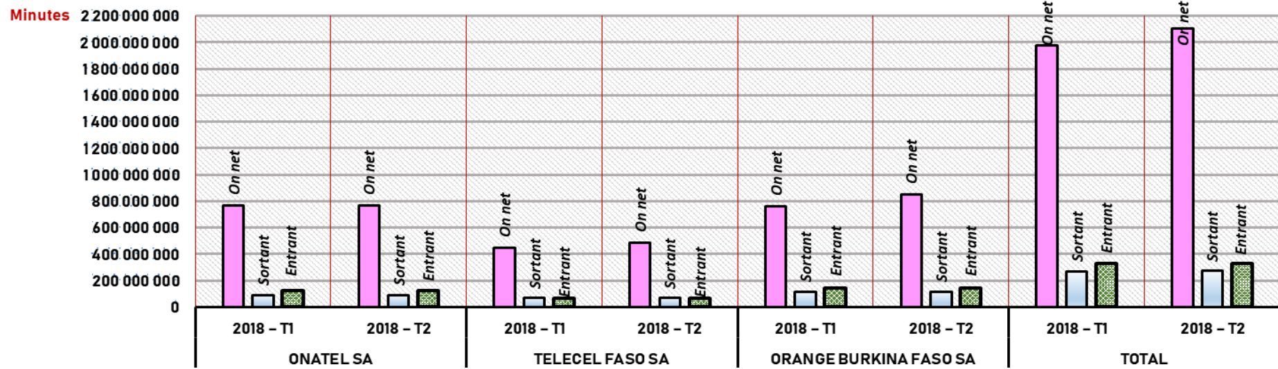
Figure 3 : Evolution des courants de trafic voix
