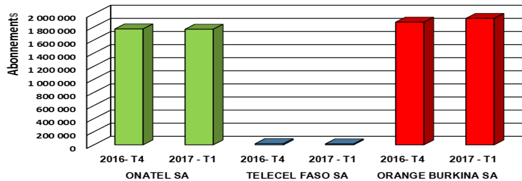
Figure 3 : Evolution du parc des utilisateurs de l'Internet sur les réseaux mobiles
