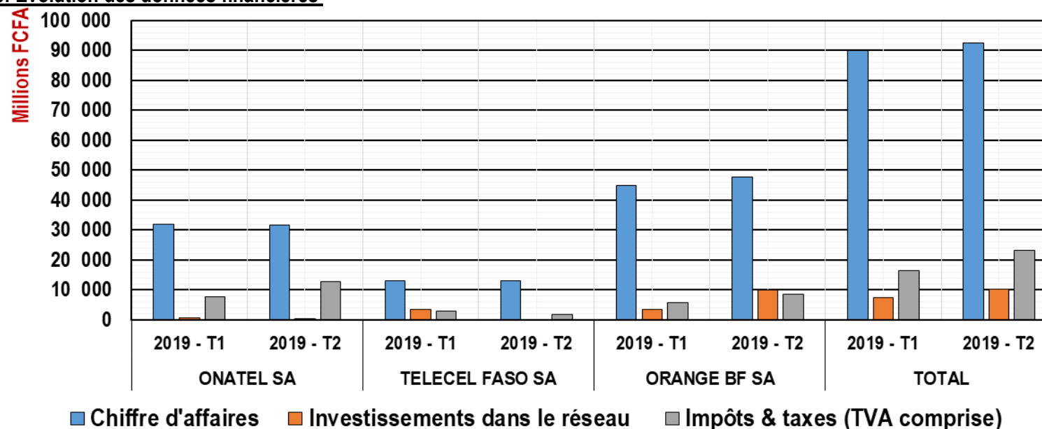
Figure 6: Evolution des données financières
